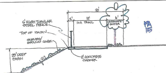
SECTION D-D
